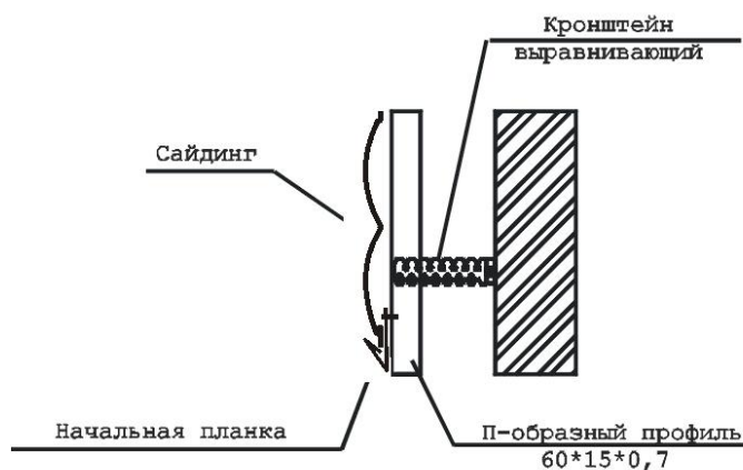
Рис. 3. Установка стартовой/финишной планки при горизонтальном монтаже сайдинга.
