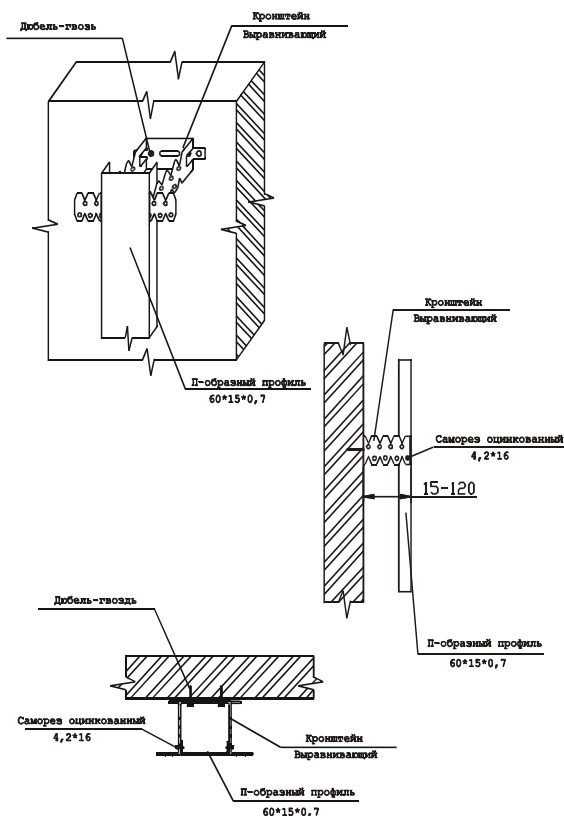
Рис. 2. Выравнивающая система
