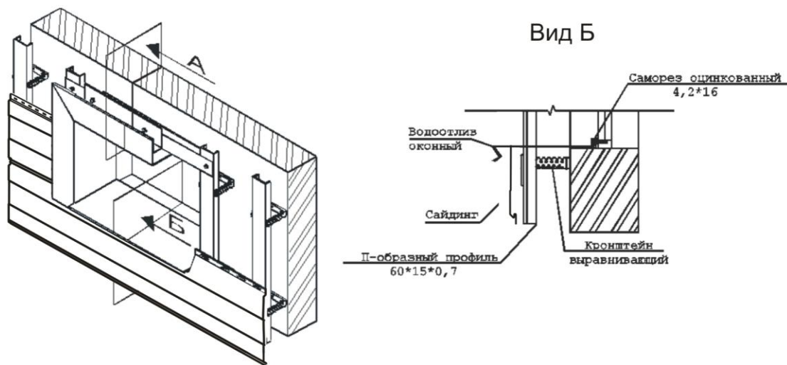
Рис 5. Обрамление оконного проема планкой внешнего откоса.
