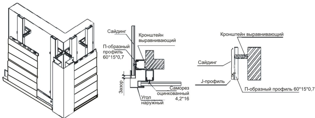
Рис. 7. Установка панелей
