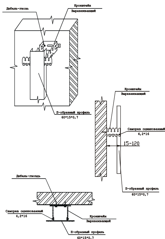
Рис. 2. Выравнивающая система
