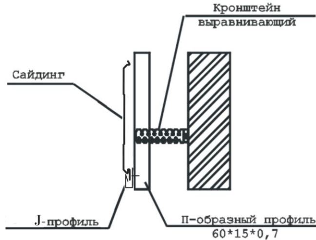
Рис. 3. Установка J-профиля при горизонтальном монтаже сайдинга.
