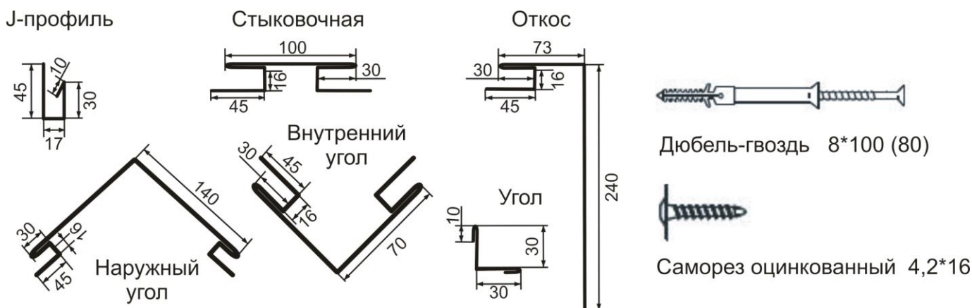
Рис. 1 Комплектующие
