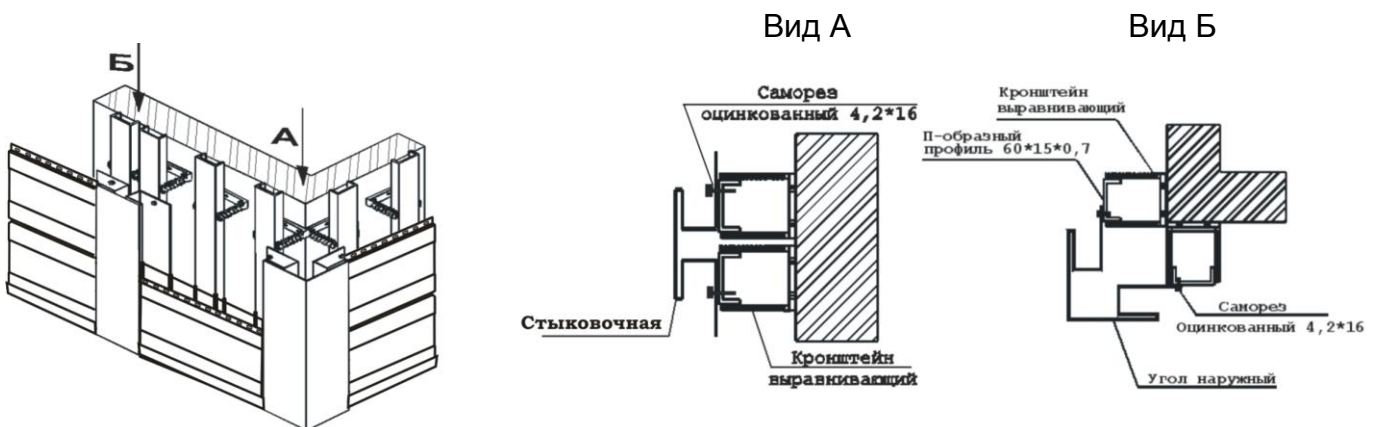
Рис 4. Установка углов и Н-образных планок.
